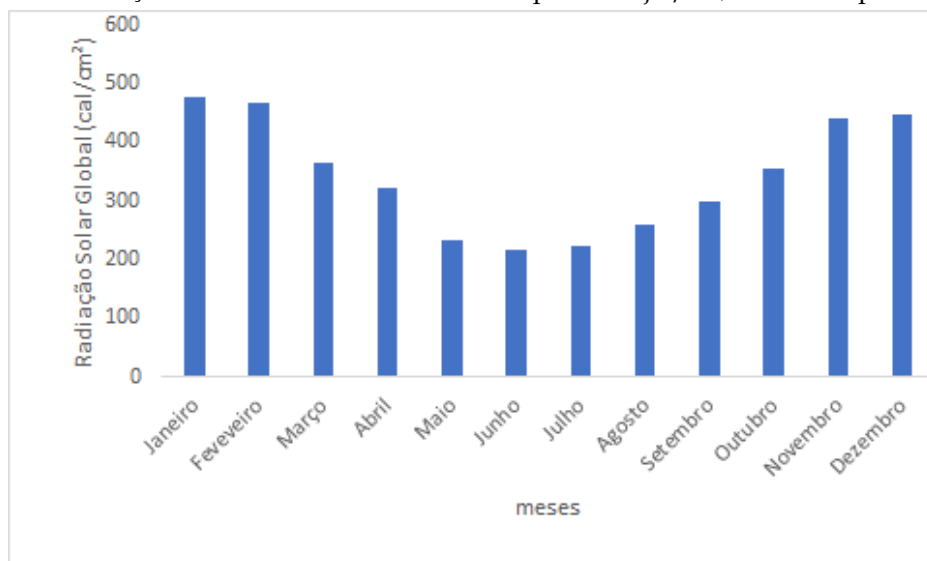
Figura 16 - Radiação Solar Global Média do Município de Itajaí/SC, referência para a região.
