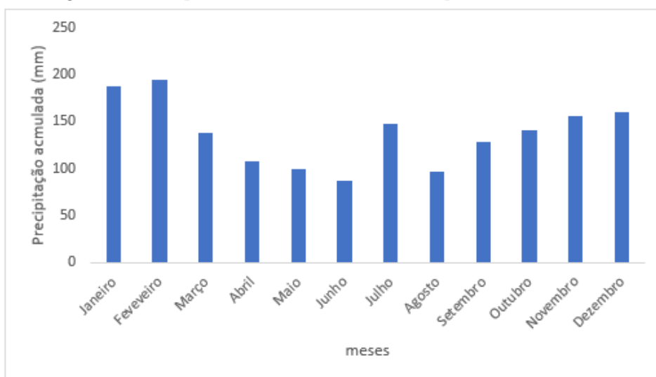
Figura 14 - Precipitação Acumuladas do Município de Camboriú/SC.
