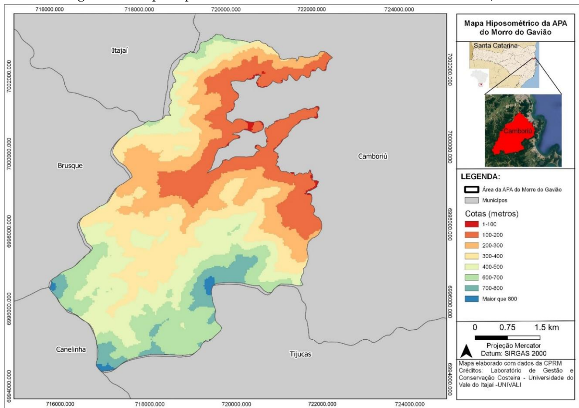
Figura 27 - Mapa Hipsométrico da APA do Morro do Gavião, Camboriú/SC.
