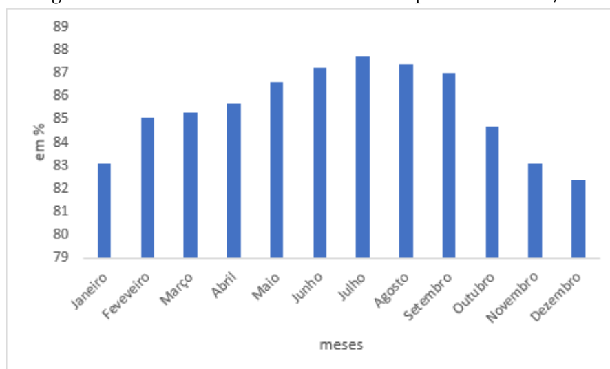
Figura 13 - Umidade Relativa do Ar do Município de Camboriú/SC.
