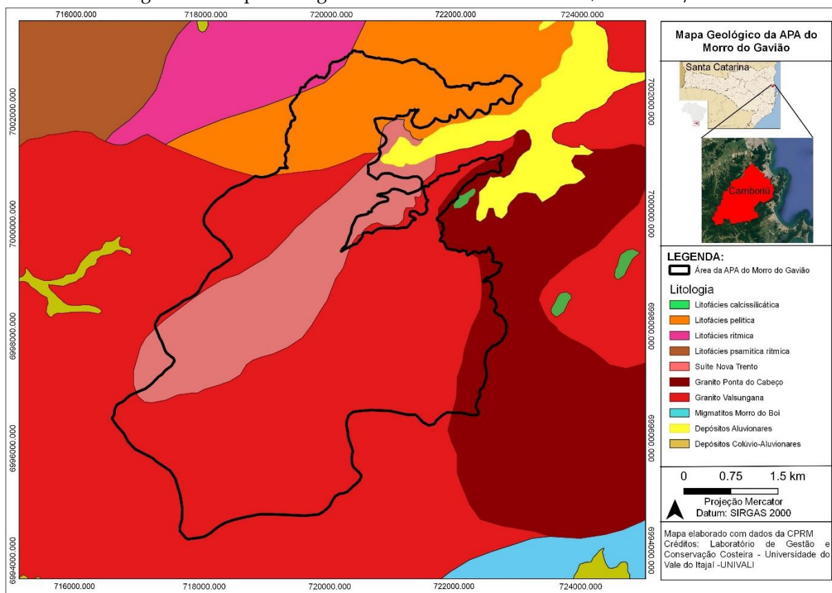
Figura 18 - Mapa Geológico da APA do Morro do Gavião, Camboriú/SC.
