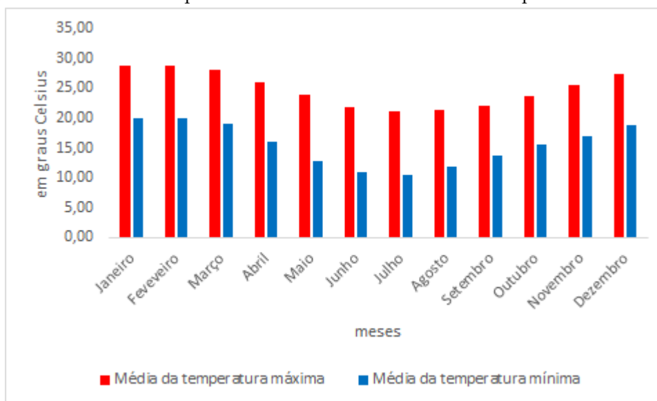
Figura 11 - Média da Temperatura Mínima e da Máxima do Município de Camboriú/SC.
